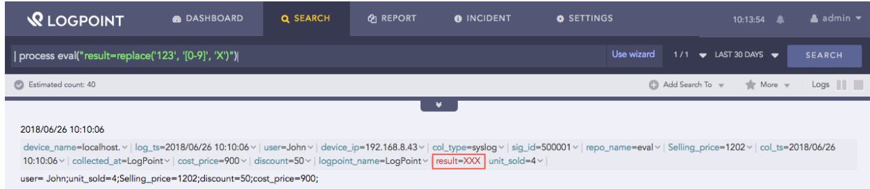
Fig. 8: Replace function
