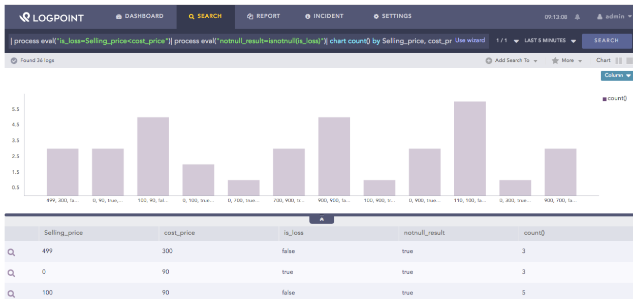
Fig. 3: Isnotnull function
