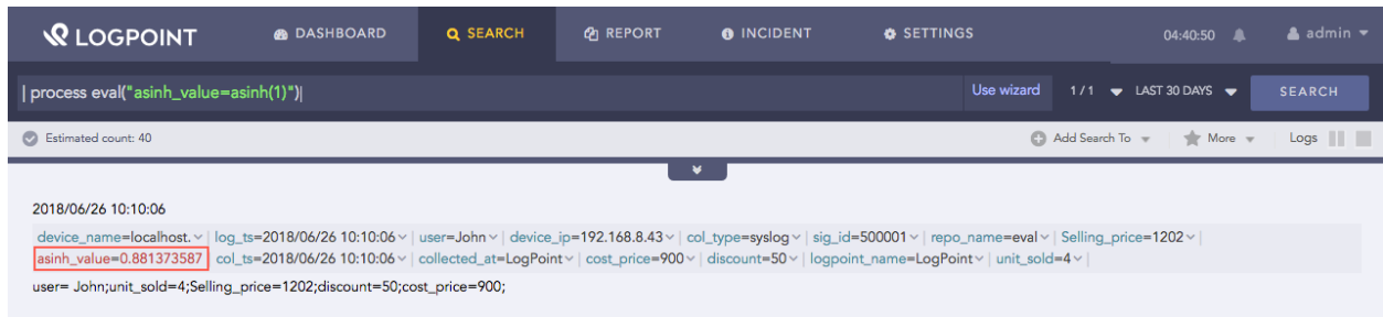
Fig. 4: Asinh function
