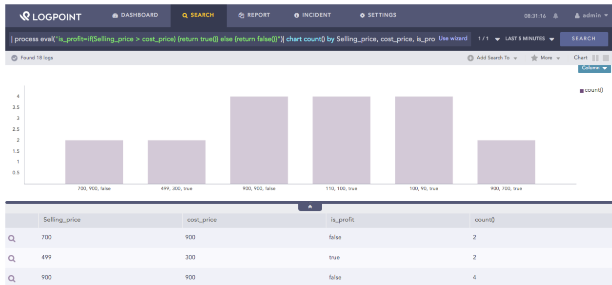
Fig. 7: False function
