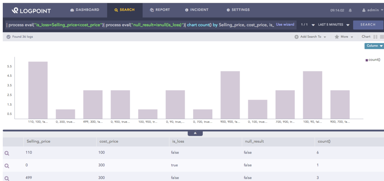
Fig. 4: Isnull function
